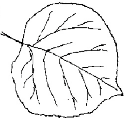
LIME
